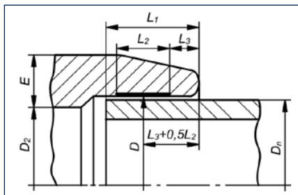
Рис. 2. Геометрия фитинга
